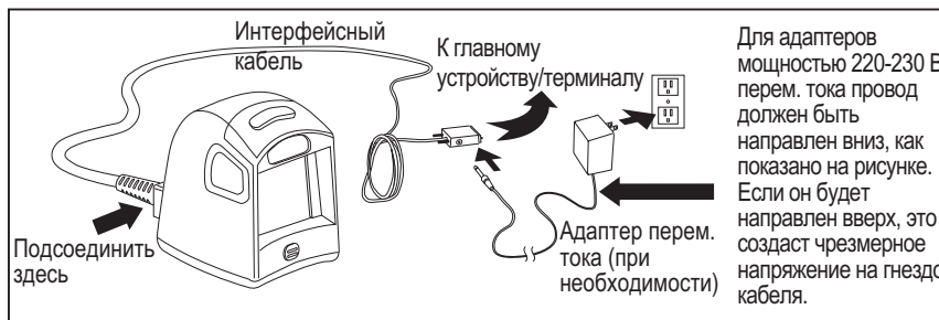
Рис. 1. Последовательное подключение RS-232 или USB-подключение с помощью адаптера переменного тока
