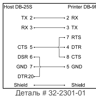
Компьютер DB-25S Принтер DB-9P
